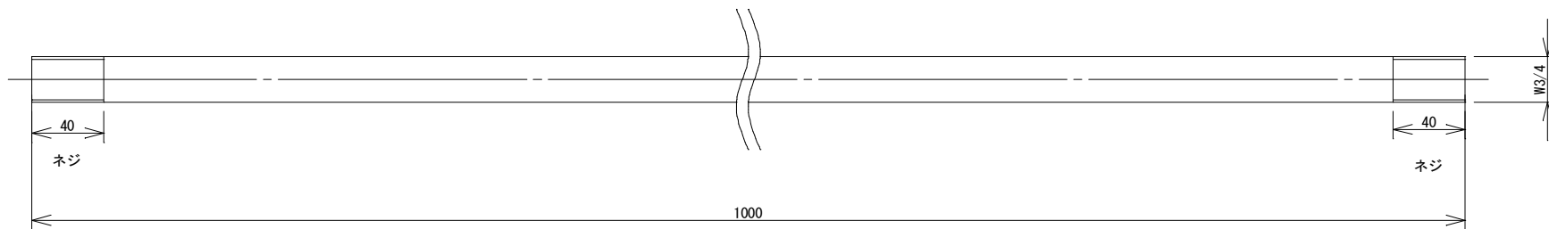
両ネジロッド (φ19×1000)
