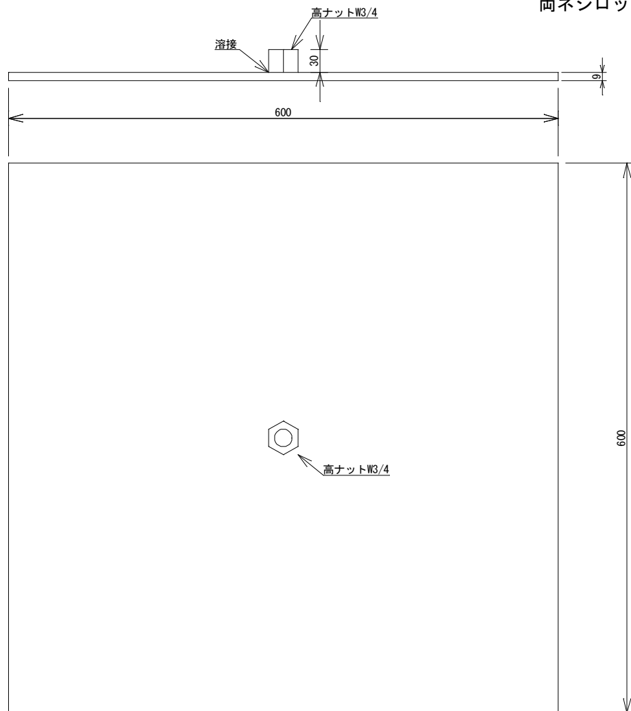
沈下板 (600×600×9)
