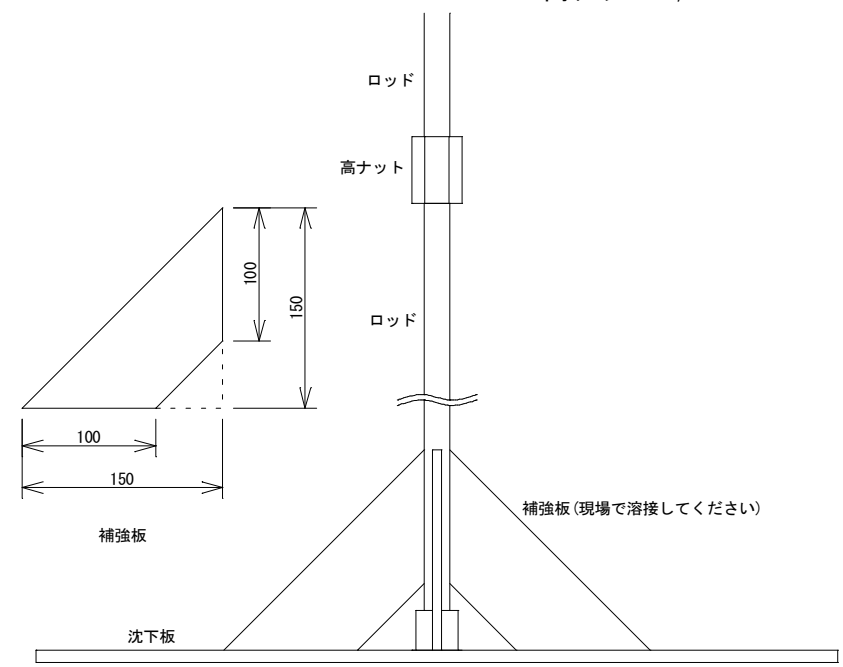
組立図
