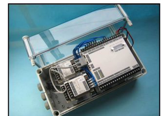
計測ボックスへの組込例(4CH 収納)
